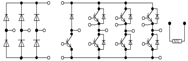
等效电路图
