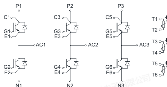
等效电路图
